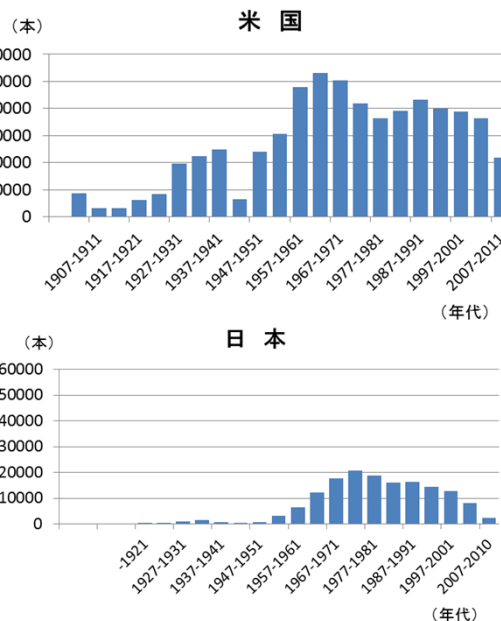
(グラフ2) 日・米 建築年代別の橋梁数
